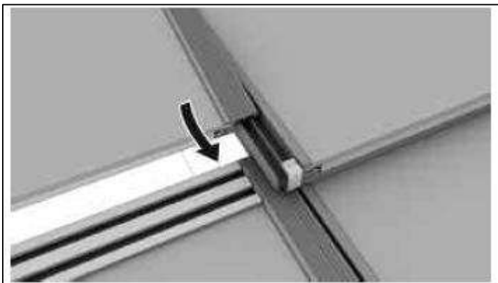
Figura 4-13: montaggio moduli
