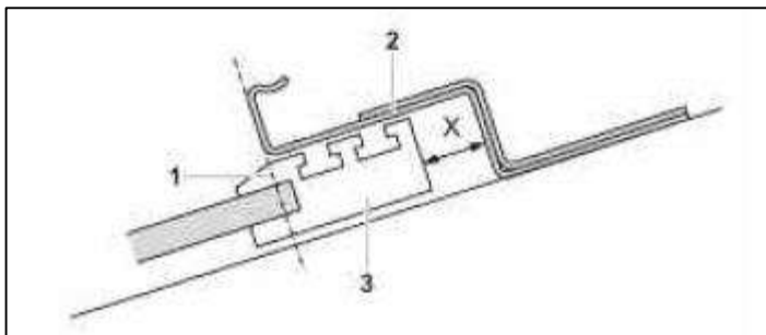
Figura 4-11: distanza fra staffa di montaggio e modulo
