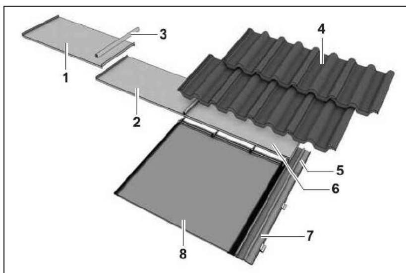
Figura 3-13: lamiere di raccordo superiori
