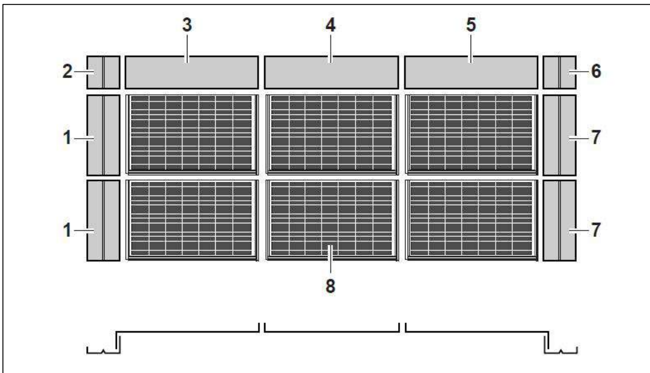
Figura 3-8 montaggio delle lamiere di raccordo
