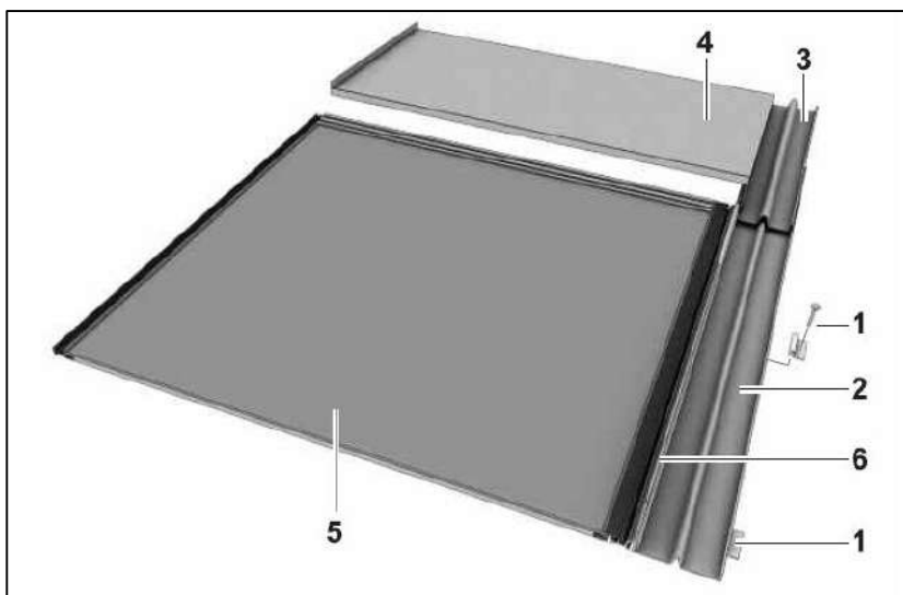
Figura 3-11: lamiera di raccordo laterale superiore destra
