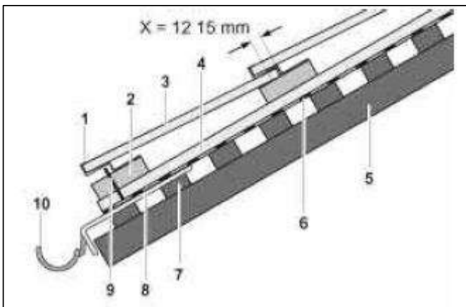
Figura 4-4 Collegamento a tetto direttamente su grondaia
