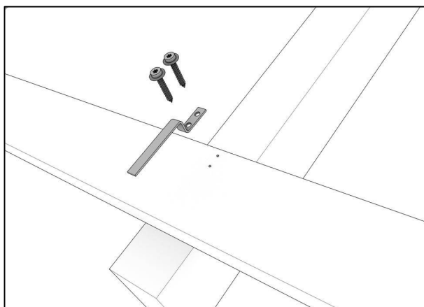
Figura 3-4: Staffa di montaggio "vetro"
